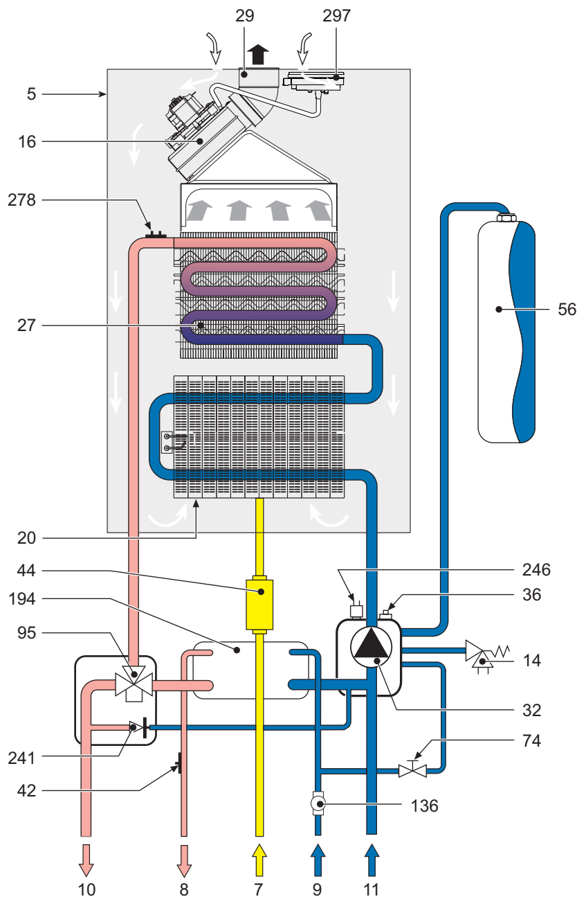
fig. 34 - Circuito idraulico
