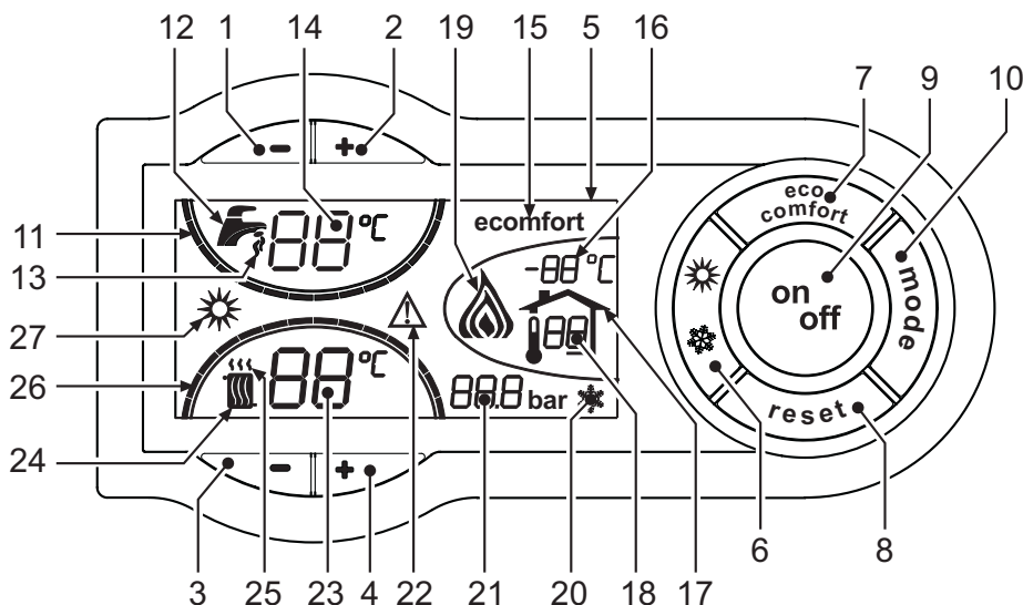
fig. 1 - Pannello di controllo
