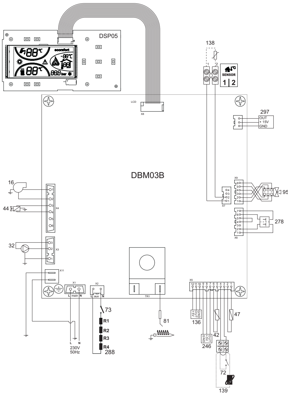
fig. 35 - Schema elettrico
