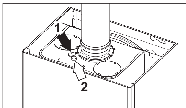
fig. 31 - Analisi fumi
