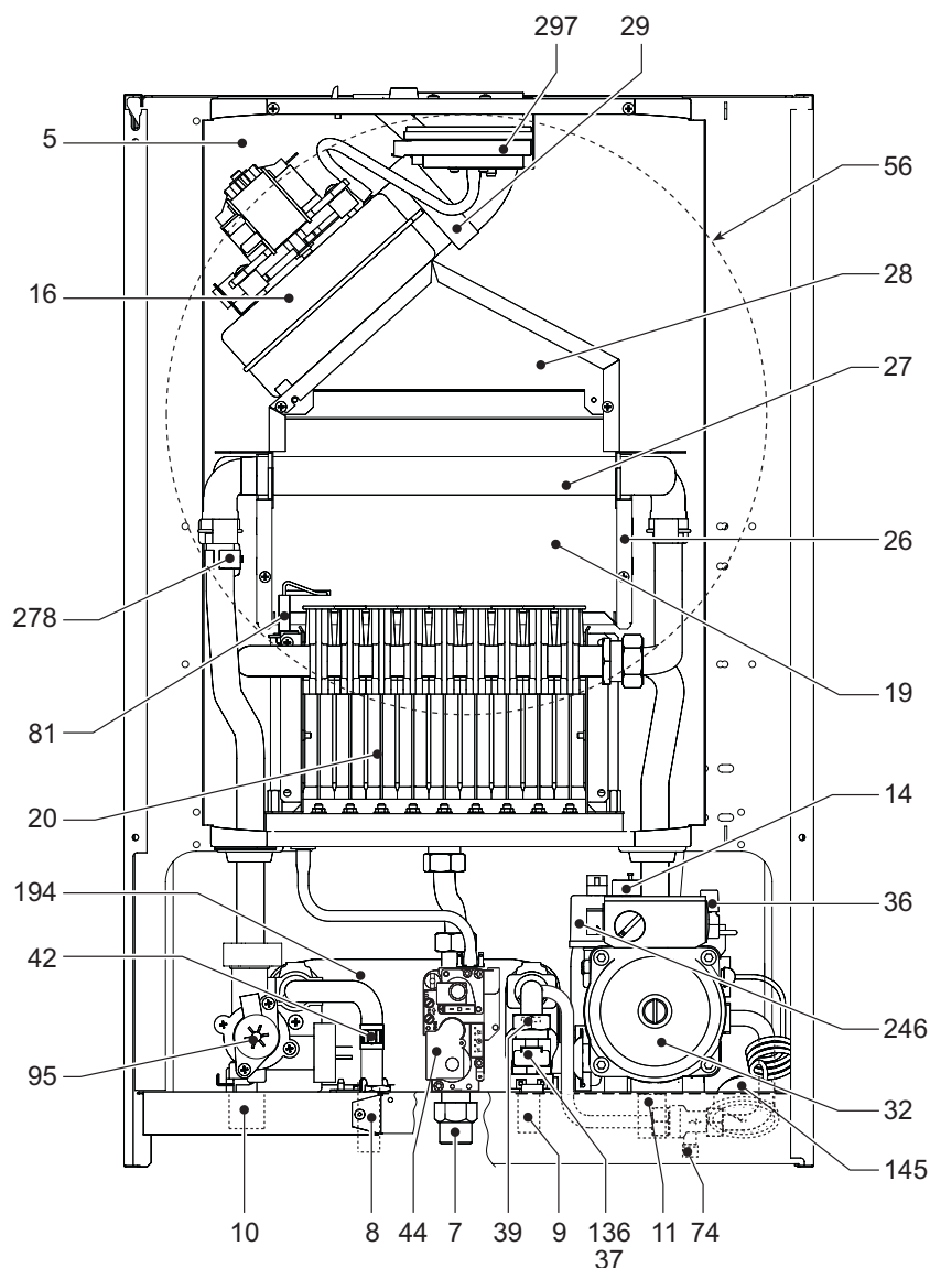
fig. 33 - Vista generale
